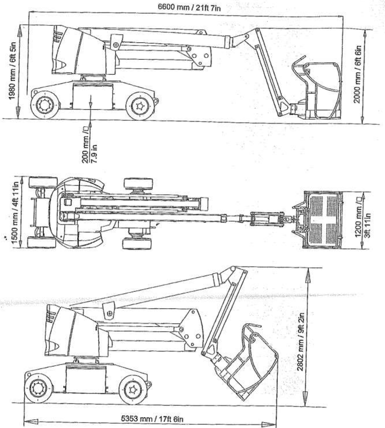
Fig. 5 - Ingombri HA15IP
